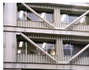
耐震用ブレース Earthquake- proof braces
